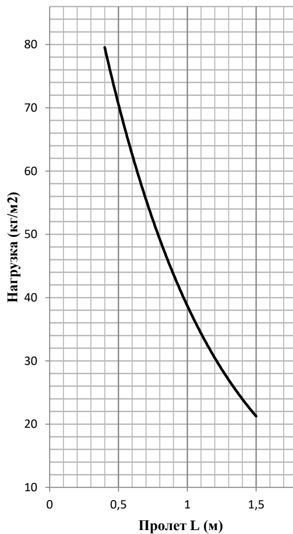
330 16-5 S Нагрузка на отрыв
