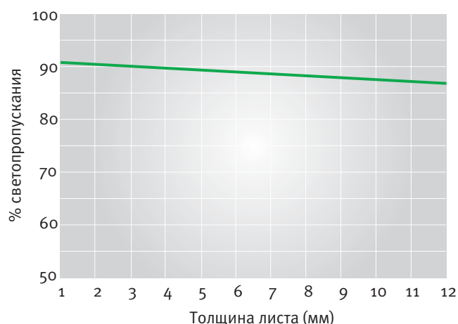
График 2. Коэффициент светопропускания полимерного стекла Novattro® относительно толщины листа
