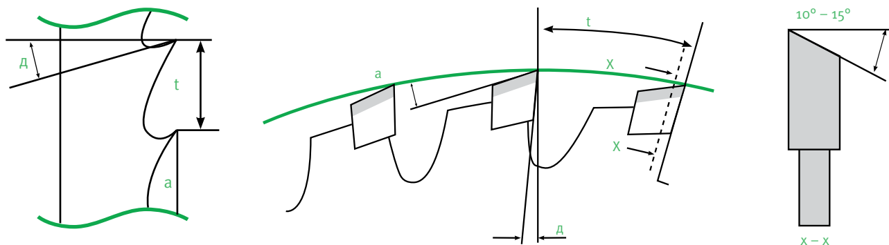
Рисунок 1. Ленточная пила и дисковая пила
