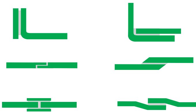
Рисунок 5. Рекомендуемые конструкции соединений
