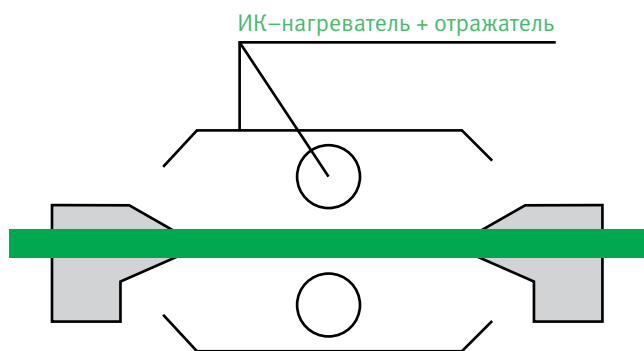
Рисунок 5. Горячий линейный изгиб. Стекло Novattro® должны местно нагреваться с помощью ИК-излучателей или провода сопротивления.
