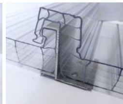
На пересечении с прогонами Анкер для 25 мм арт. 494025 НЧП-7625 ОБ
