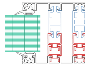
Уплотнитель ТЭП арт. 902904 СТП-252
