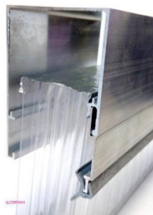
Профиль верхний для 40 мм (U, S) арт. 420080 НЧП-8013
