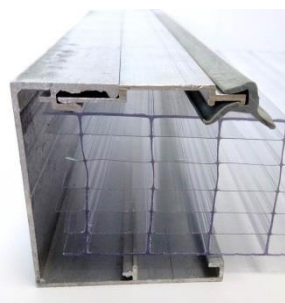
Профиль рамный для 40 мм (U, S) арт. 420040 НЧП-7620
