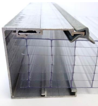
Профиль рамный для 40 мм (U, S)
