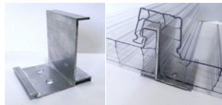
На пересечении с прогонами Анкер для 25 мм арт. 494025 НЧП-7625 ОБ
