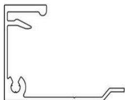
Профиль боковой для 25 мм арт. 462540 НЧП-8292
