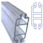
Термоадаптер (ПК) арт. 361661
