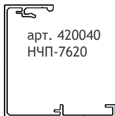
Профиль рамный для 40 мм (U, S)
