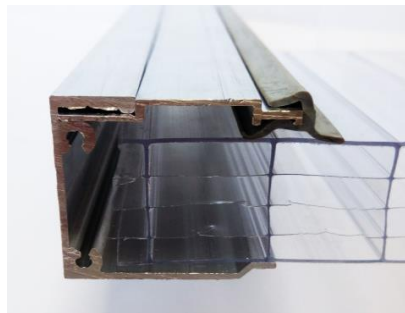
Профиль боковой для 25 мм арт. 462540 НЧП-8292
