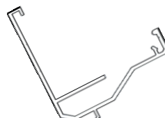
Профиль нижний наклонный для 40-S мм арт. 404051 НЧП-8024
