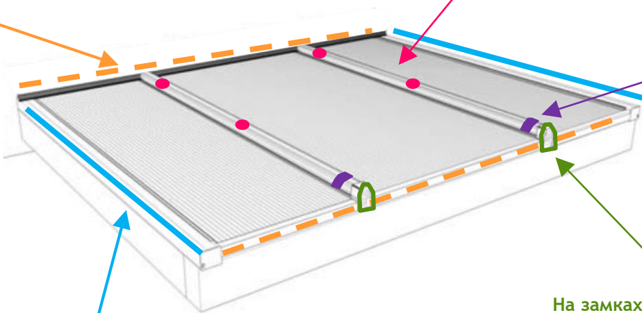
Профиль торцевой для 25 мм арт. 462511 НЧП-7627
