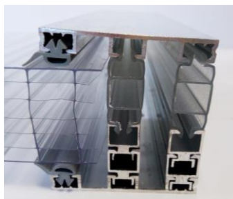
Термопрофиль универс. арт. 460060 НЧП-7621
