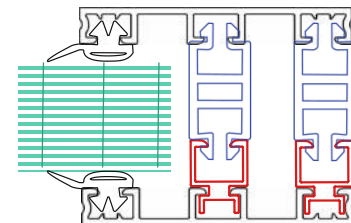
Уплотнитель ТЭП арт. 902904 СТП-252
