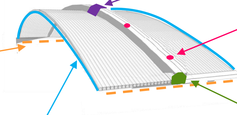
На пересечении с прогонами Анкер для 25 мм арт. 494025 НЧП-7625 ОБ
