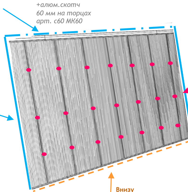
Профиль нижний наклонный для 40-S мм арт. 404051 НЧП-8024
